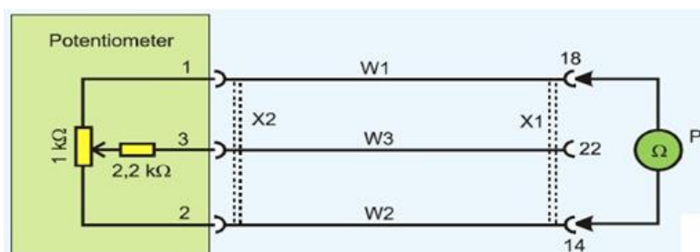
Mérési elrendezés az irányítóegység csatlakozótól mérve
