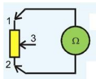
Potenciométer ellenállásmérés
