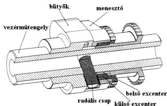
Lengőbütökös szelepvezérlő rendszer
