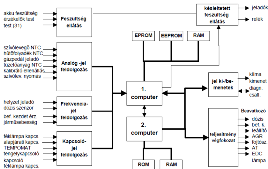
A DCU 1 irányítóegység blokkvázlata
