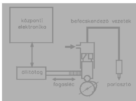
EDC „él” vezérlésű soros adagolón
