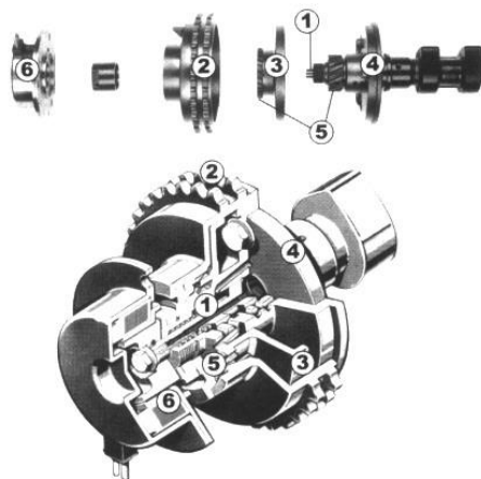
A Mercedes változtatható szívószelep vezérlése (1. vezérlődugattyú, 2. lánckerék, 3. tolőhüvely, 4. a vezérműtengely válla, 5. ferde fogazat, 6. elektromágnes)
