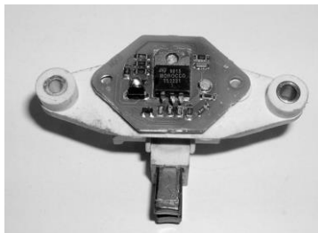
Elektronikus integrált áramkörös kivitelben készült, kefetartóval egybeépített feszültségszabályzó
