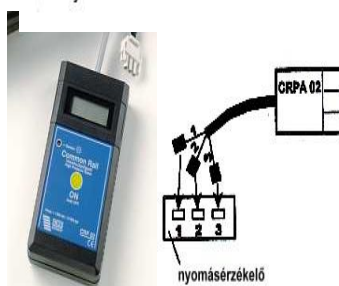
Digitális nyomásmérés
