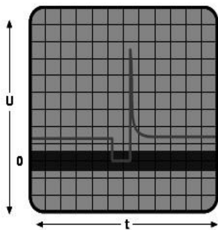
Befecskendező szelep
