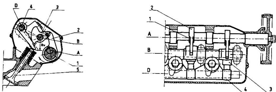
Torazza-féle lengőbütykös vezérlés
