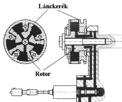
Szárnylapátos elven működő vezérműtengely-állító egység
