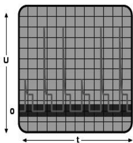
Aktívszén-szűrő szelep mágnesszelep
