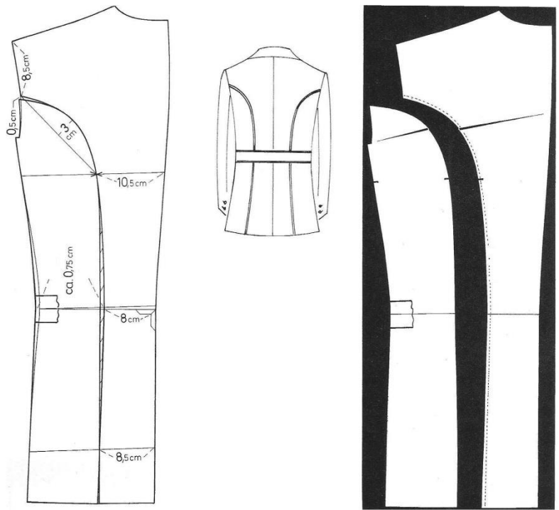
100. ábra Sportzakó háta modellezés3
