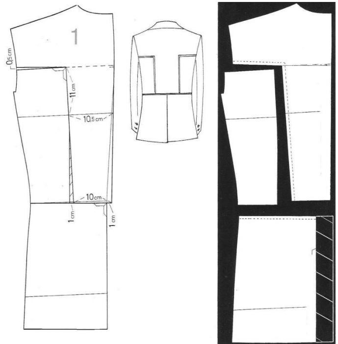
101. ábra Sportzakó háta modellezés4
