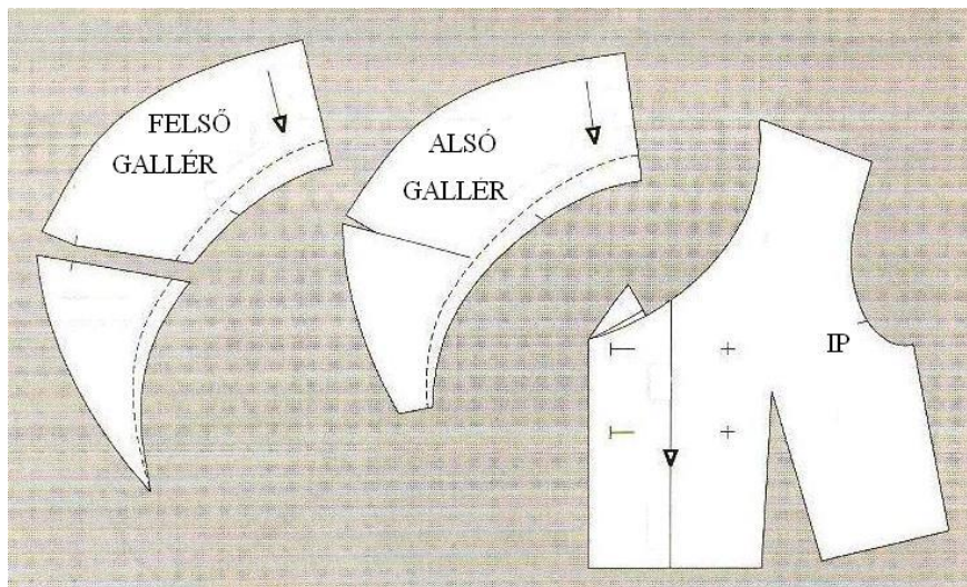
39. ábra Hátrész illesztése gallér alampintái
