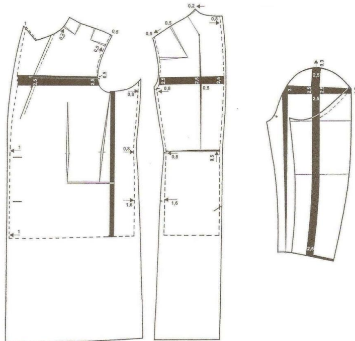
103. ábra Zakó minta átalakítási lehetőségei
