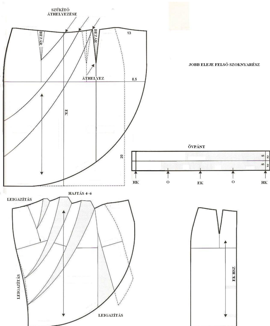
28. ábra Szoknya modellezése
