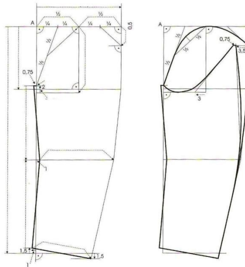
83. ábra Ujja szerkesztés
