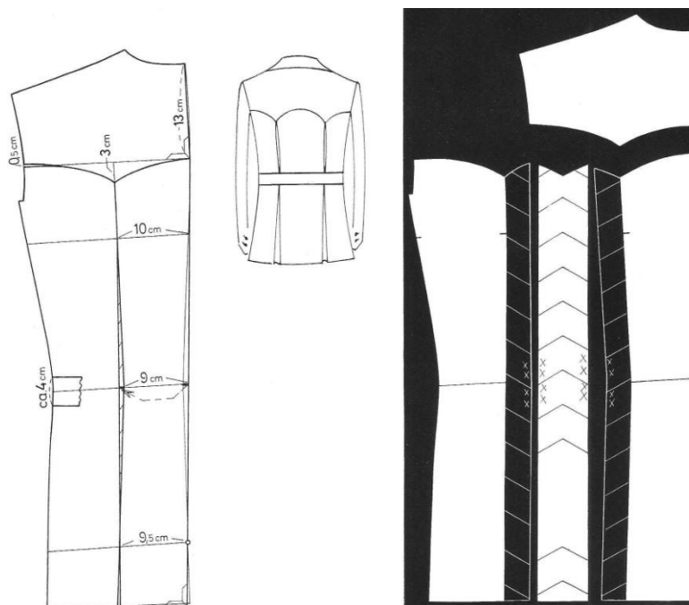
99. ábra Sportzakó háta modellezés2
