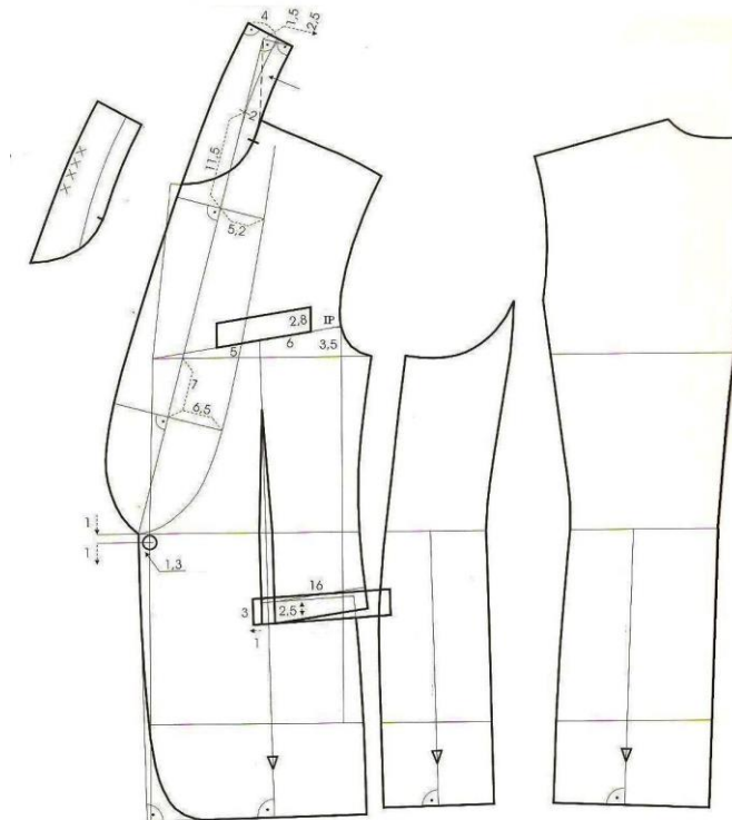
93. ábra Szmoking alapmintái
