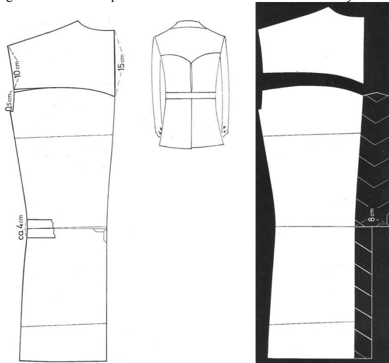
98. ábra Sportzakó háta modellezés1
