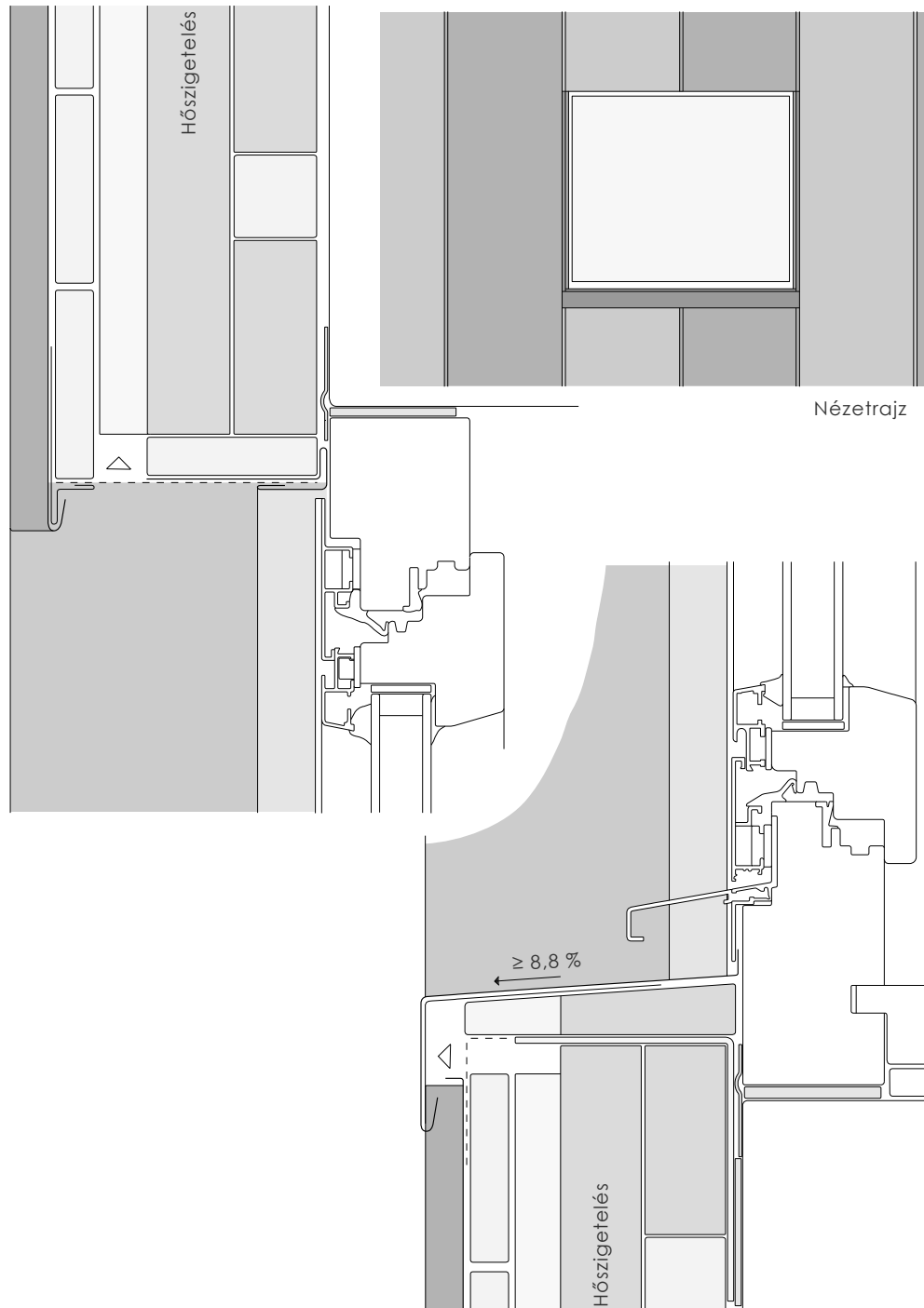
Homlokzati nyílások beépítése (5.1 ábra)
