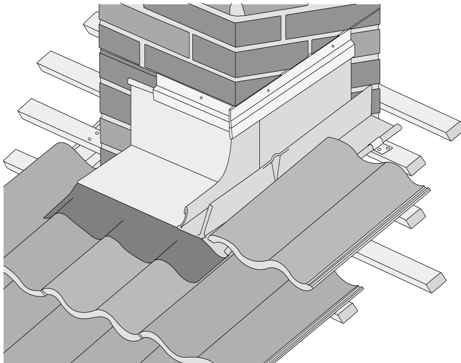
3.8 ábra Ólombetétes kéményszegély nagyalakos cserépfedésben
