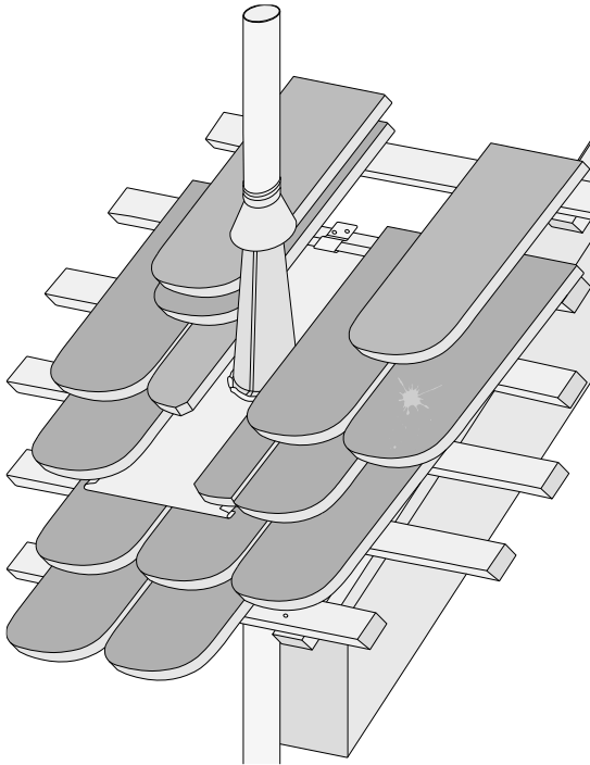
3.11 ábra Rúdátvezetés cserépfedésű tetőben
