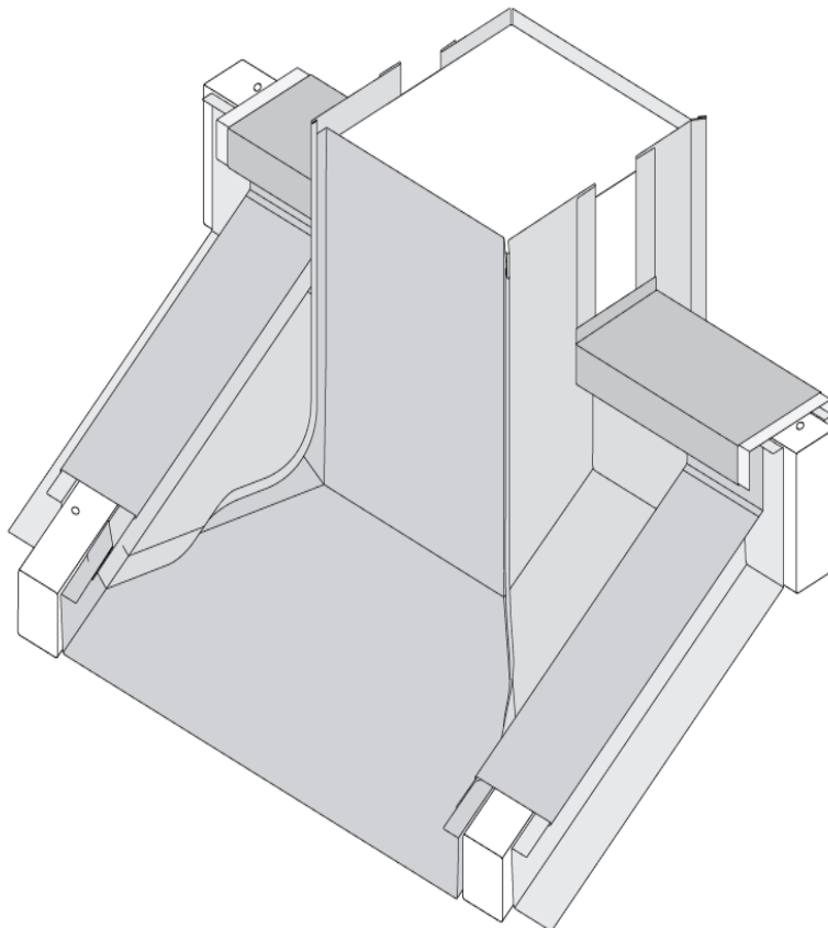
4.35 ábra Kéményszegélyezés lécbetétes fedésben
