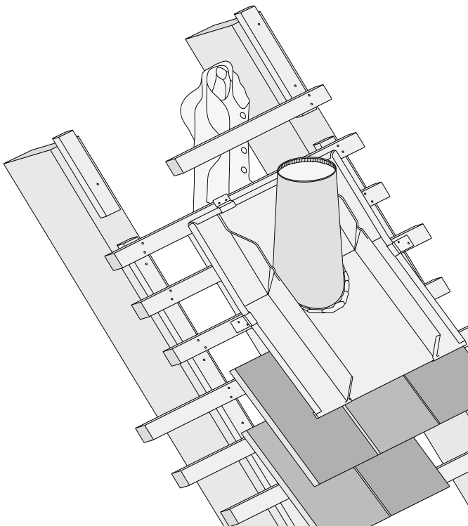
3.12 ábra Szellőzőcső kivezetés cserépfedésű tetőben
