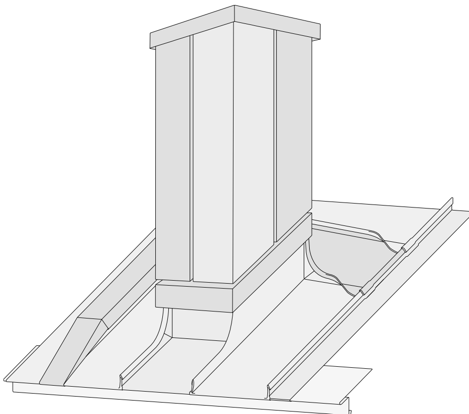
5.5 ábra: Kéményburkolat csaphornyos elemekkel
