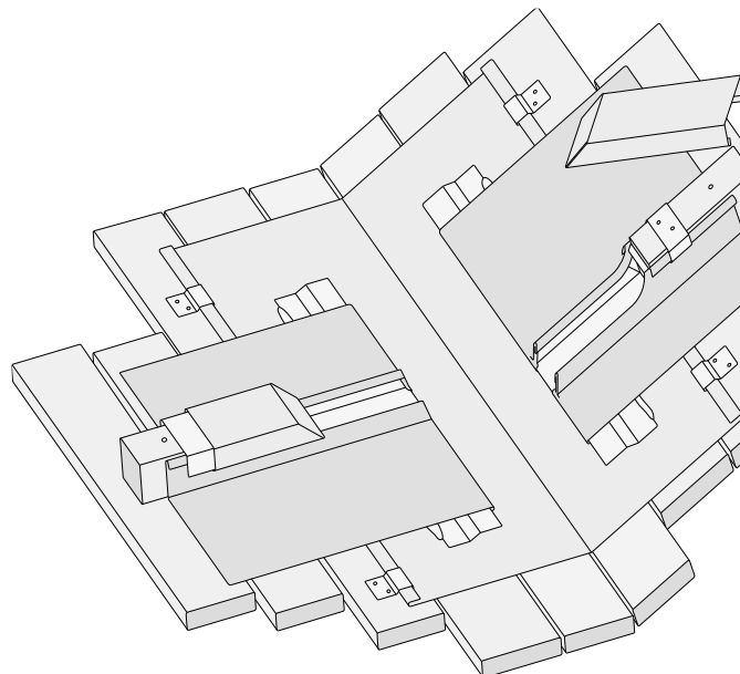
4.32 ábra Lécbetétes fedés vápakialakítása, ráforrasztott rögzítő egyszeres, fekvőkorccal (lejtése \geq 10^\circ )
