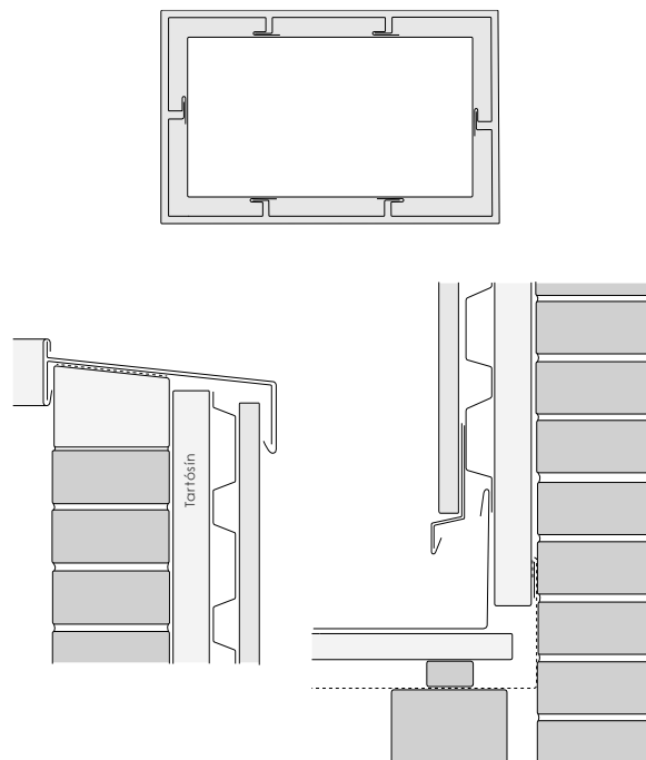
5.4 ábra: Kéményburkolat csaphornyos elemekkel készült burkolattal háttérvázon, alsó és felső csomópont
