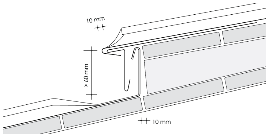
c) lejtéslépcső (4.11 ábra)
