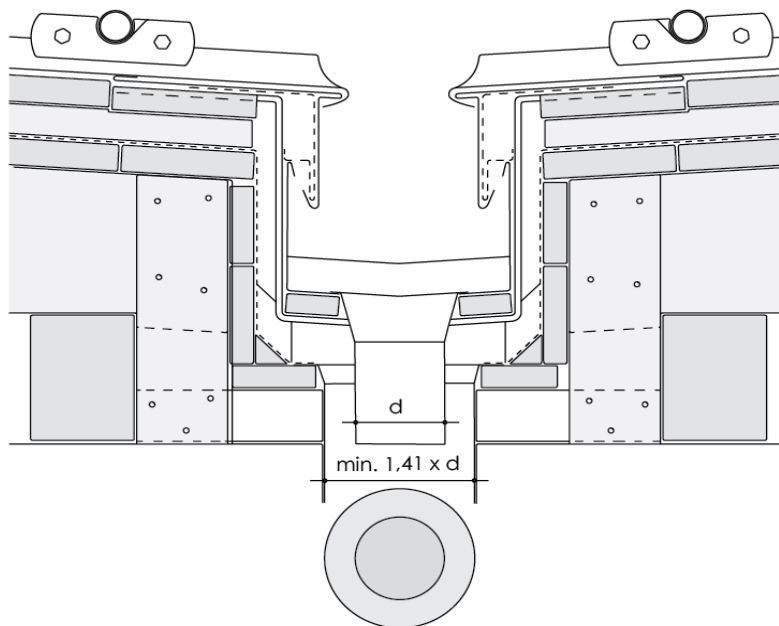
1.5 ábra Belső helyzetű csatorna, kétszintű vízelvezetéssel
