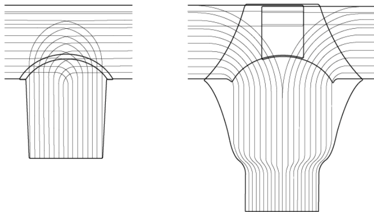
1.1 ábra A hengeres formájú és a tölcséres összefolyó hidrodinamikai viselkedése: Az előbbinél a lefolyócső keresztmetszetének mindössze 70 %-a vehető számításba
