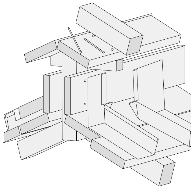
4.34 ábra Gerincszellőző kialakítása lécbetétes fedésben
