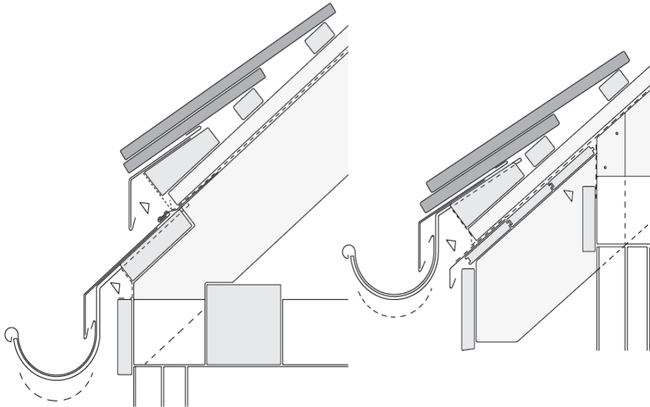
1.3 ábra A homlokzati síktól nem előreugró és előreugró ereszt, függő ereszcsonnával. A második vízvezető réteg a csatornába, illetve az alatt van kivezetve
