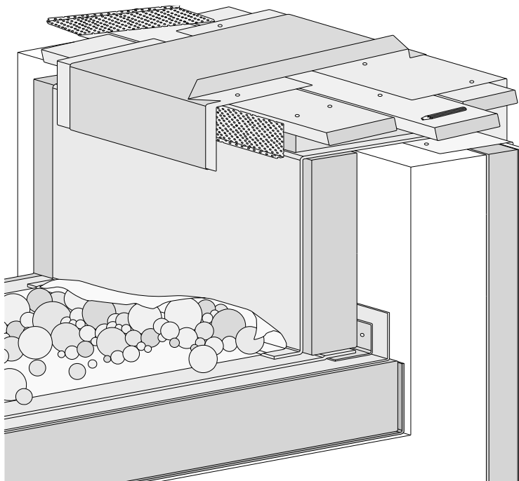
2.4 ábra Attikafal-szegély kialakítása PVC szigetelésű lapostetőben
