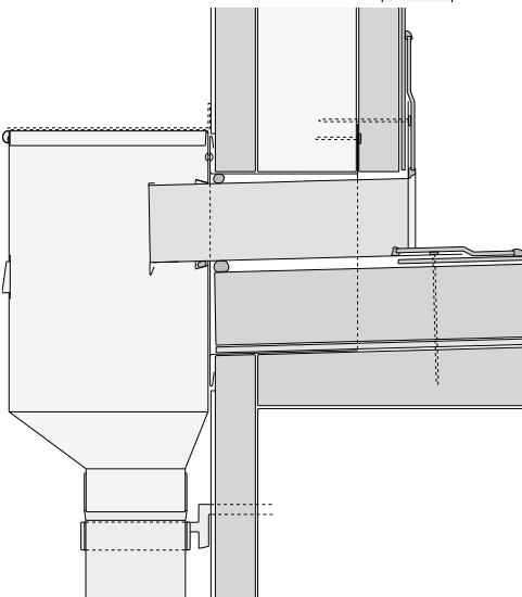
1.8 ábra Lefolyó-csatlakozás vízgyűjtő üsttel attikafalon kivezetett kifolyóhoz lágyfedésű tetőben
