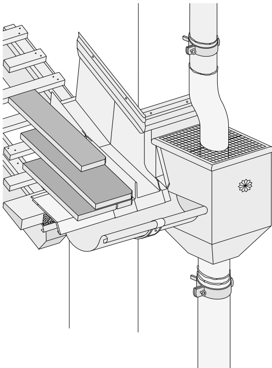
1.7 ábra Lefolyócsatlakozás vízgyűjtőüsttel cserépfedésű tetőben
