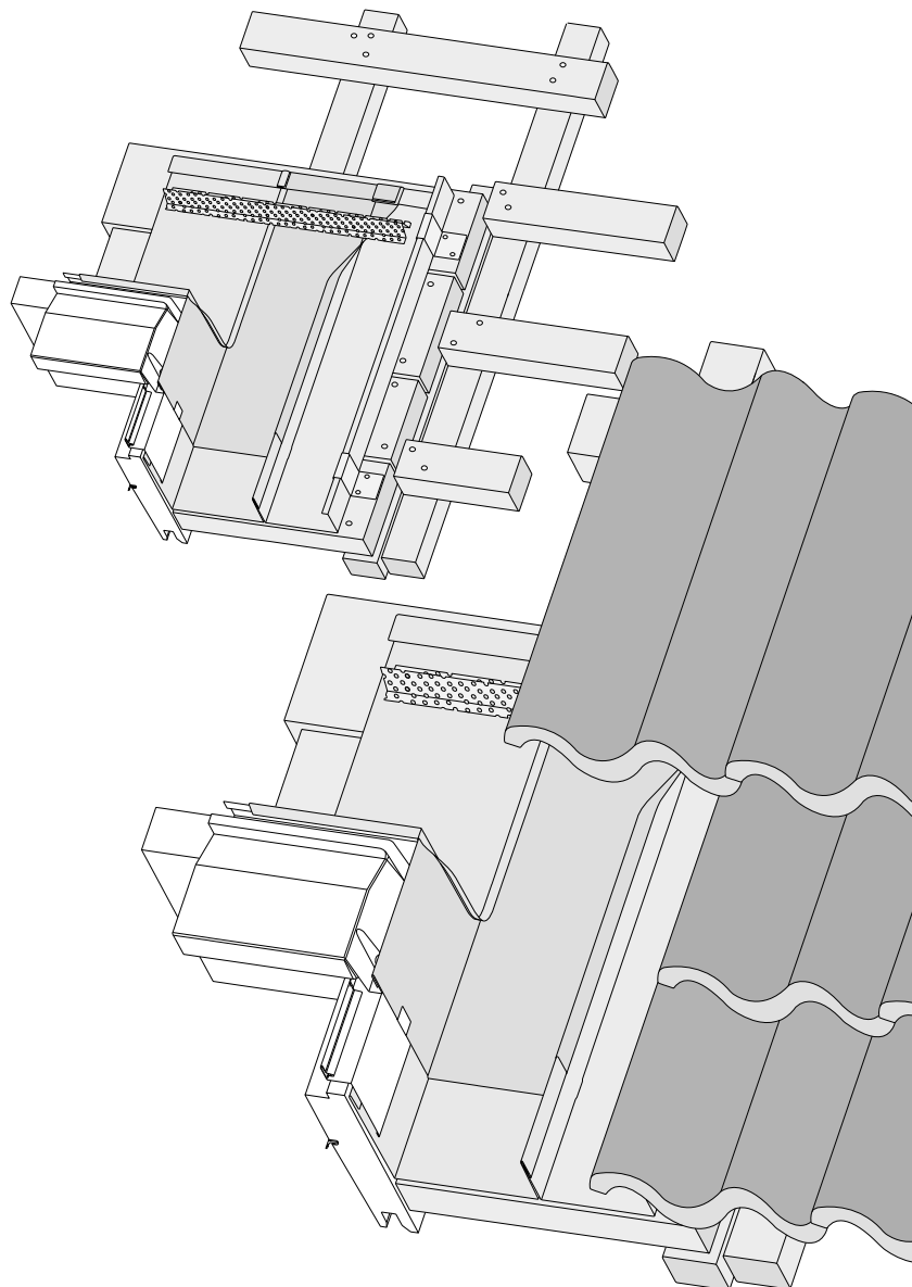
3.9 ábra Tetősíkablak egyedi szegélyezése cserépfedésű tetőben
