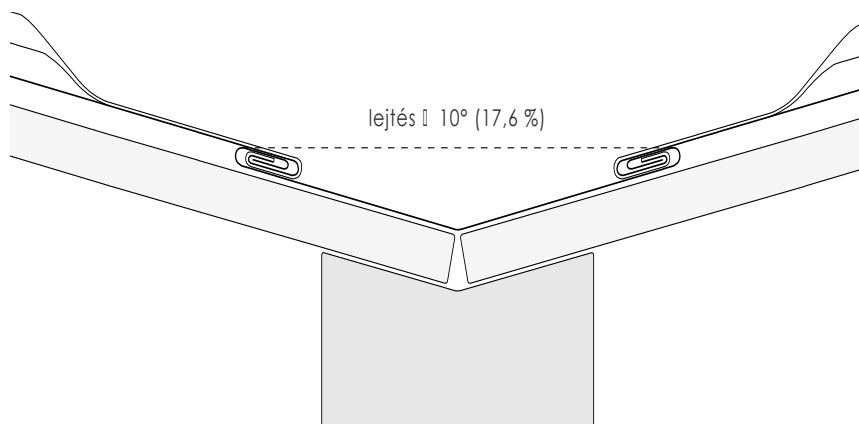
4.23 ábra Vápakialakítás két oldalról kétszeres fekvőkorccal
