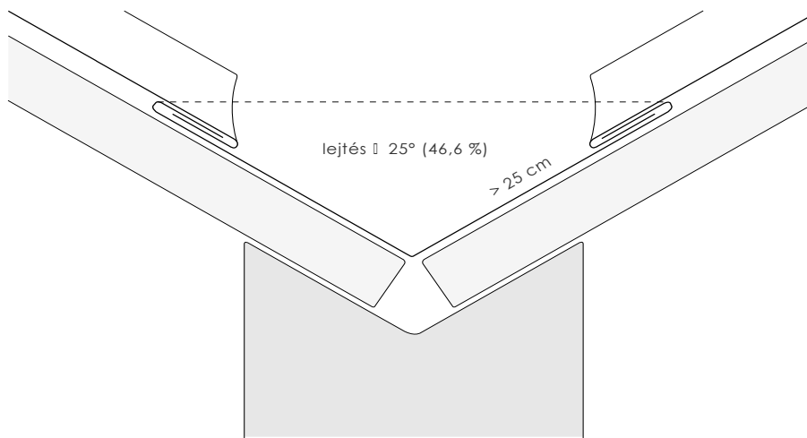
4.18 ábra Vápakialakítás két oldalról egyszeres fekvőkorccal
