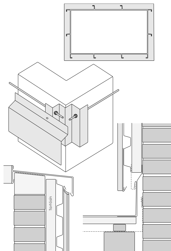
5.3 ábra: Kéményburkolat állókorcos fedéssel, fém aljzaton és tartóelemekkel, metszet, alsó és felső csomópont
