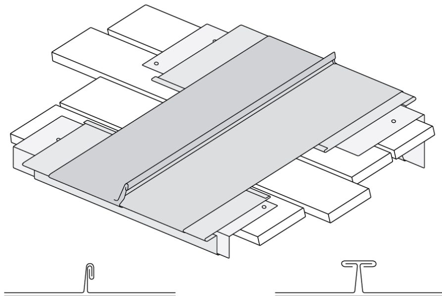
2.7 ábra Letakarások állókorccal kialakított dilatációs kapcsolatai
