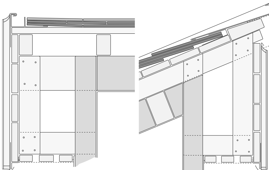
3.3 ábra Korcolt oromfedések kiselemes fedésű tetőben
