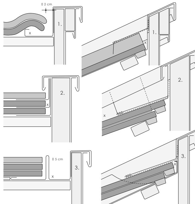
3.2 ábra Oromszegélyek kiselemes fedésű tetőben
