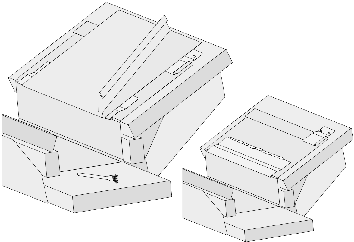
4.21 ábra: Süllyesztett vápa két oldalon a fedési ereszsávok alá is befuttatott vápalemezzel
