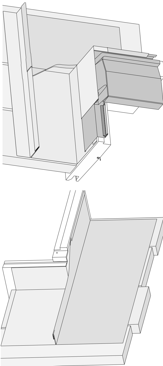
4.26 ábra Tetősikablak szegélyezési csomópontjai
