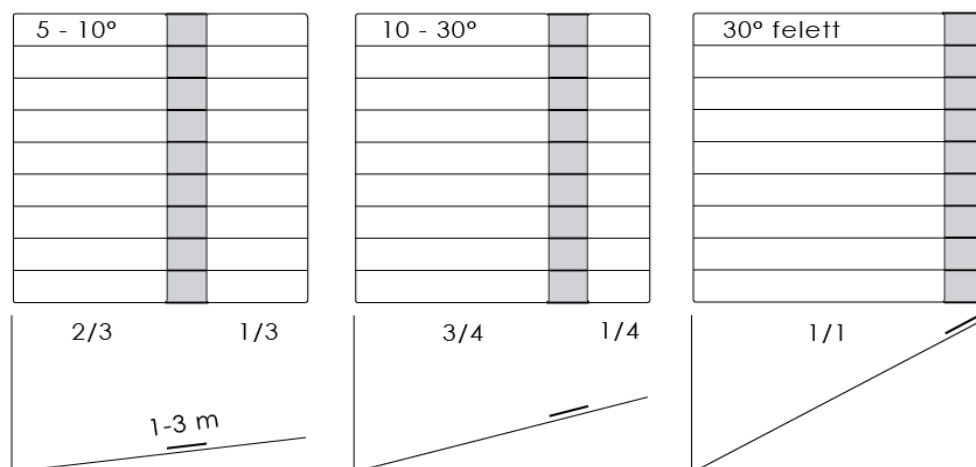
4.4 táblázat Az állófércek elrendezése a tető lejtésszögétől függően
