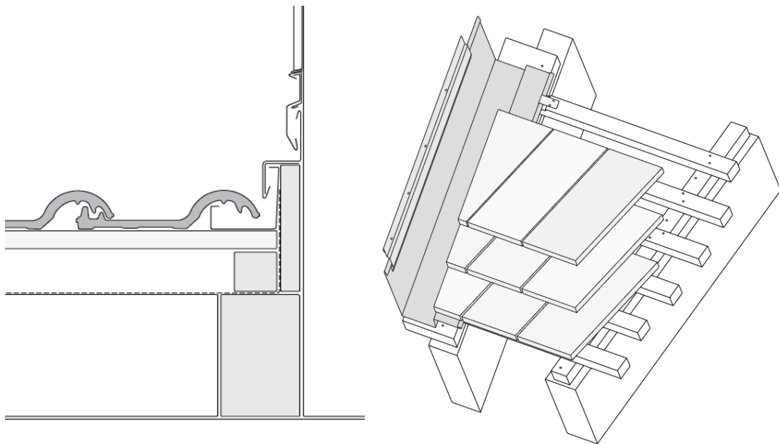
3.5 ábra Kiselemes fedésű tető falszegélyei
