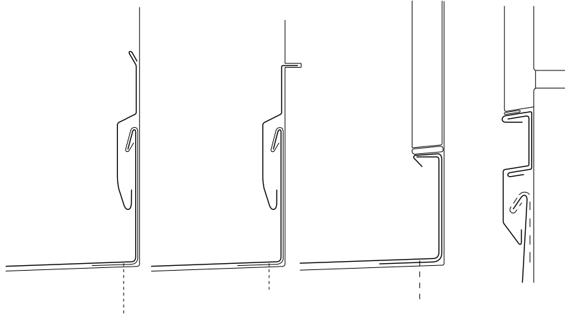
2.9 ábra Párkányok belső oldali falcsatlakozás lezárásai
