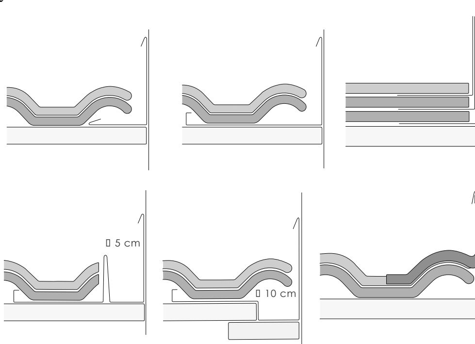
3.4 ábra Kiselemes fedésű tető falszegélyei
