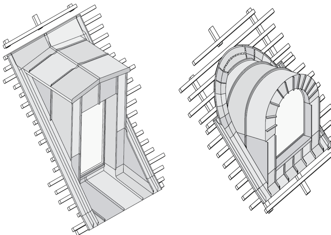
3.10 ábra A tetősíkból kiemelt tetőablakok szegélyezése
