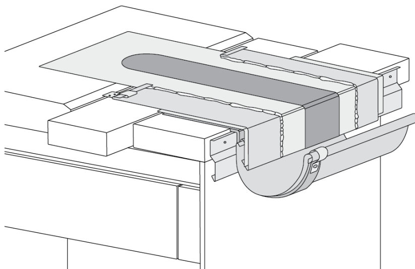
2.1 ábra Rugalmas betétes dilatációs elem, ereszszegélyben
