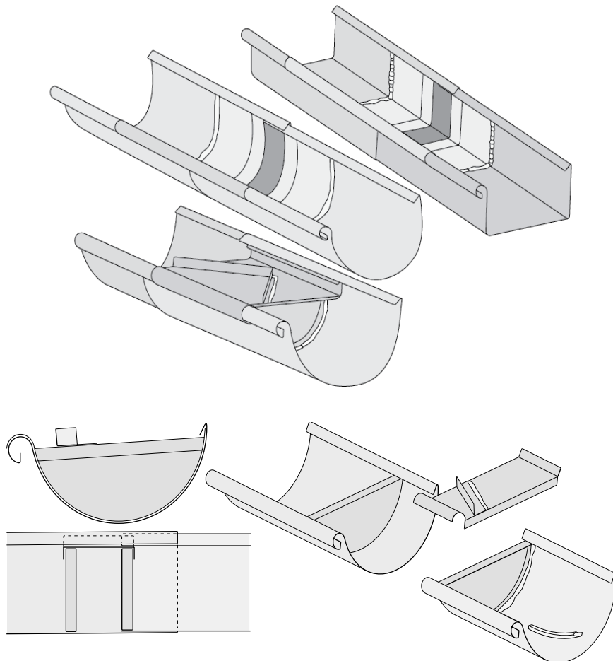
1.2. ábra Függő ereszcatorna hőmozgás-biztosításának módja
