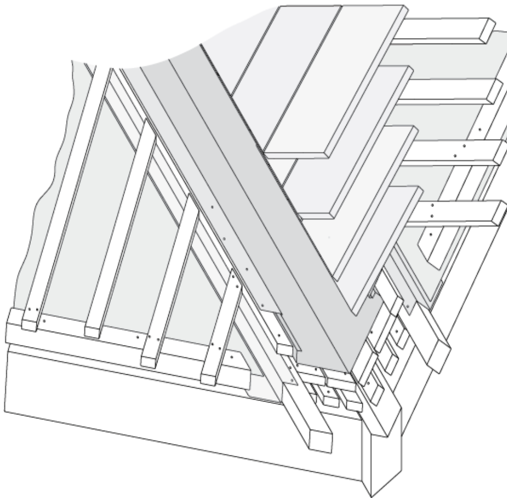
3.7 ábra Vápa-kialakítás, az alátétfőliában kialakított ferde csatornával, amely az ereszig ki van vezetve
