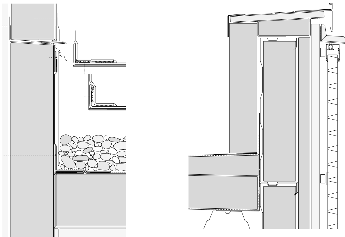
2.5 Falszegély, illetve attikafal-szegély kialakítása PVC szigetelésű lapostetőben
