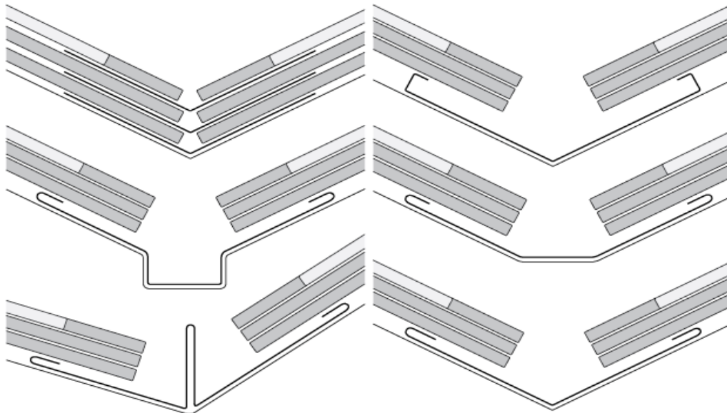
3.6 ábra Példák pikkelyfedésű magastetők vápalemezeinek kialakítására
