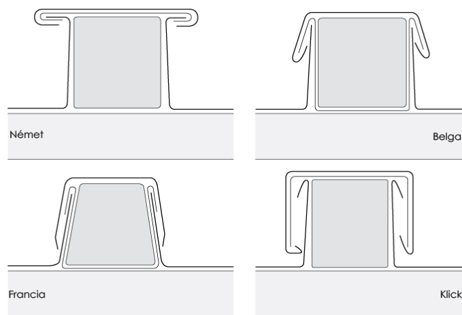
4.3 ábra A lécbetétes fedések fajtái
