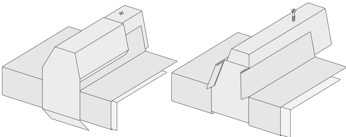
4.28 ábra francia rendszerű lécbetétes fedés ereszcsatlakozása
