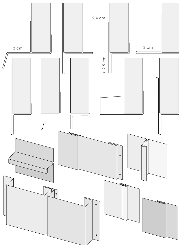
4.16 ábra Korcolt fedésű tetők oromburkolatai és fogadó szegélyei
