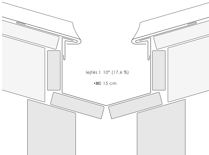
4.20 ábra Süllyesztett vápa két oldalról ereszsávval
