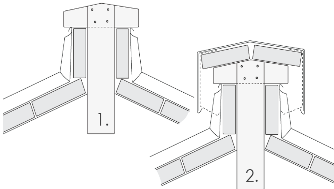
4.25 ábra Kiszellőztetett gerinc, az aljzatszerkezet megfelelő kialakításával
