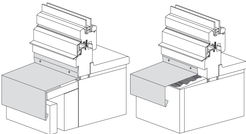
2.10 ábra Ablakpárkány-lefedés rögzítőszegéllyel és ragasztottan szerelve
