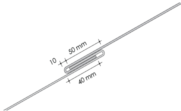
a) egyszeres fekvőkorc (4.9 ábra)
