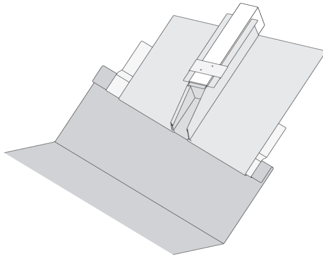
4.31 ábra Lécbetétes fedés vápakialakítása, egyszeres fekvőkorccal (lejtése \geq 25^\circ )
