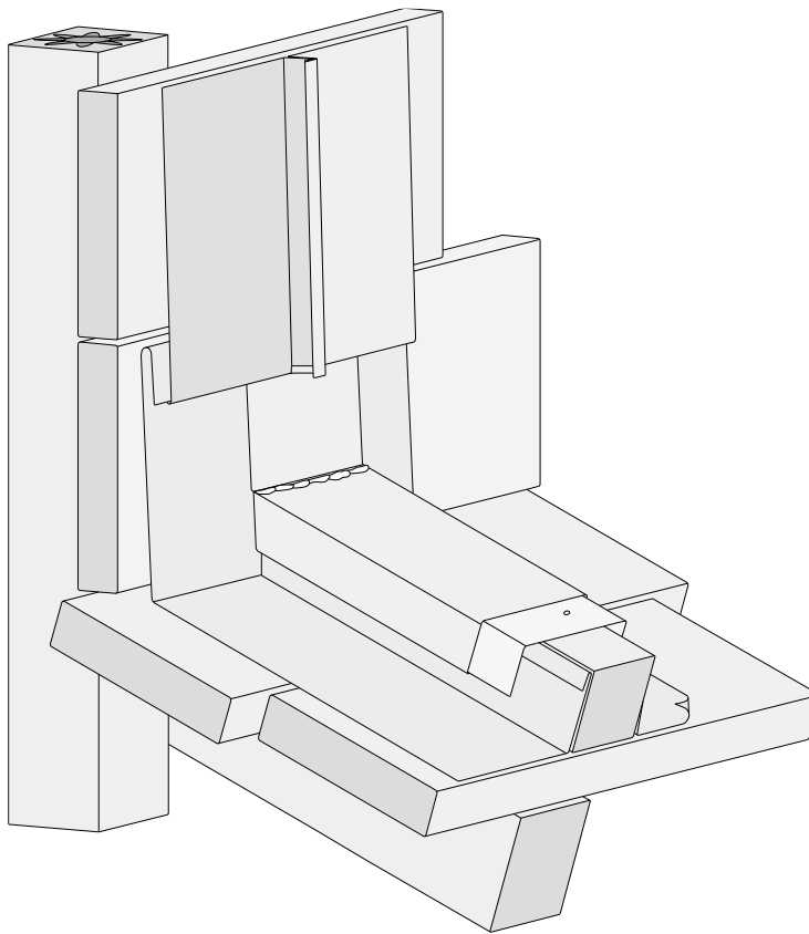
4.30 ábra A klick rendszerű lécbetétes fedés falszegély-csatlakozása
