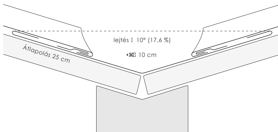
4.19 ábra Vápa két oldalról ráforrasztott rögzítősávval kialakított egyszeres fekvőkorccal
