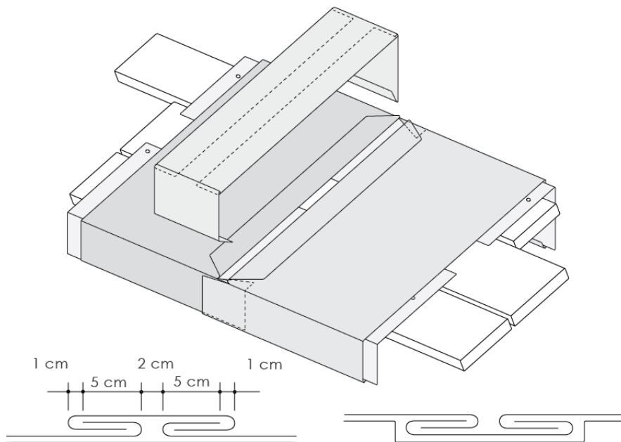
2.6 ábra Falfedési elemek hosszirányú toldása
