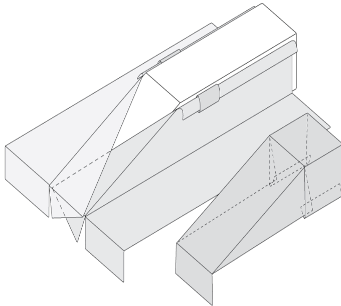
4.27 ábra Klick rendszerű lécbetétes fedés ereszcsatlakozása
