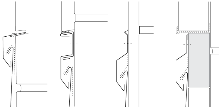
4.17 ábra A viharléc-kialakítás négy változata
