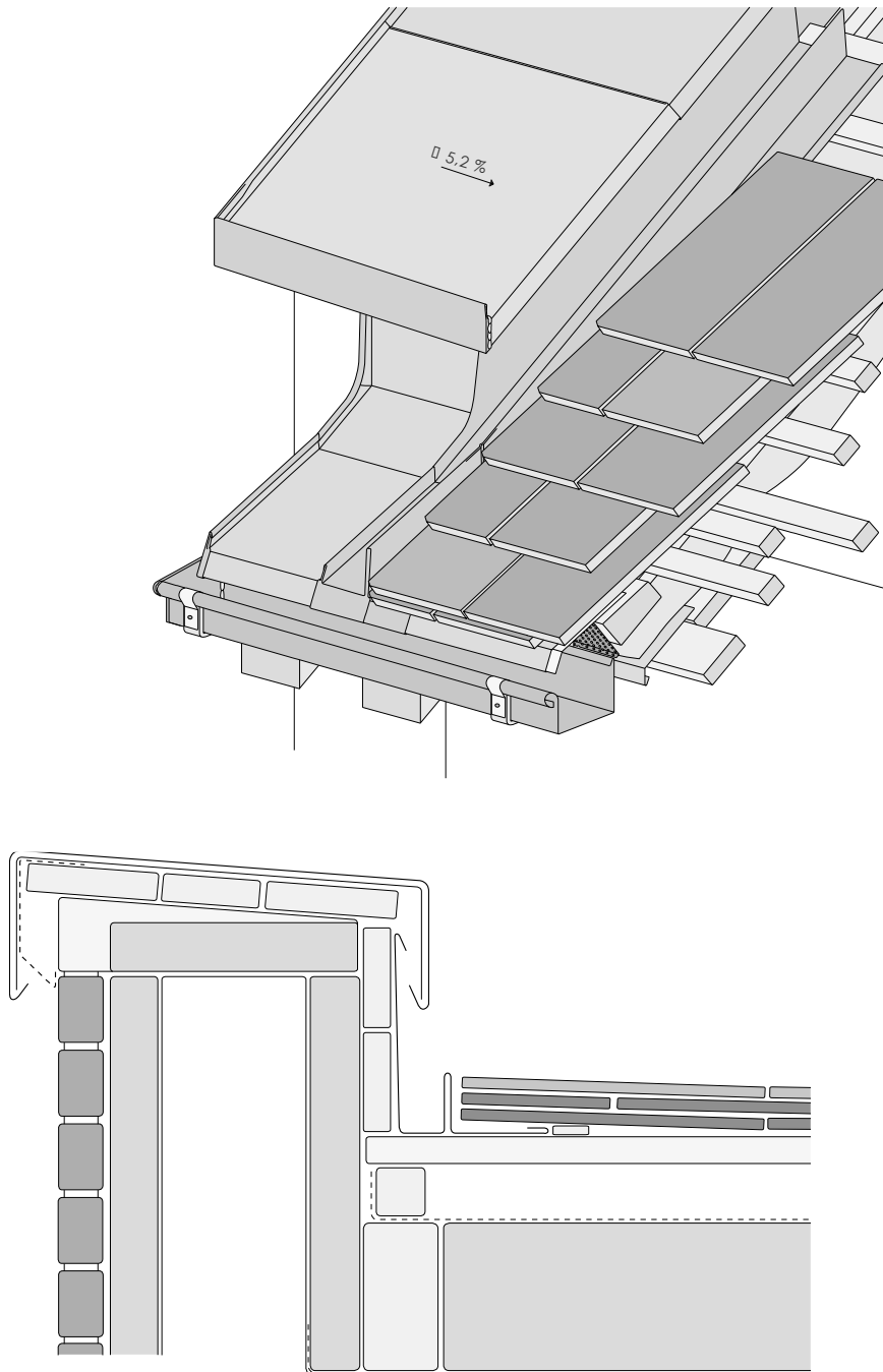
2.8 ábra Oromfal korcolt fedései
