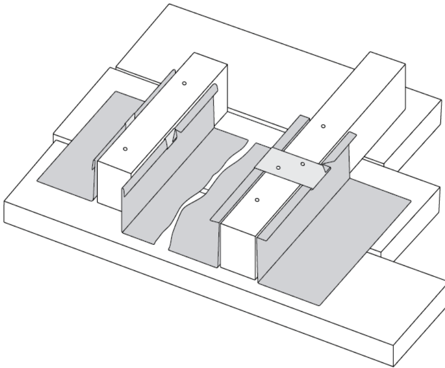
4.4 ábra Klick és német lécbetétes fedés fix rögzítése
