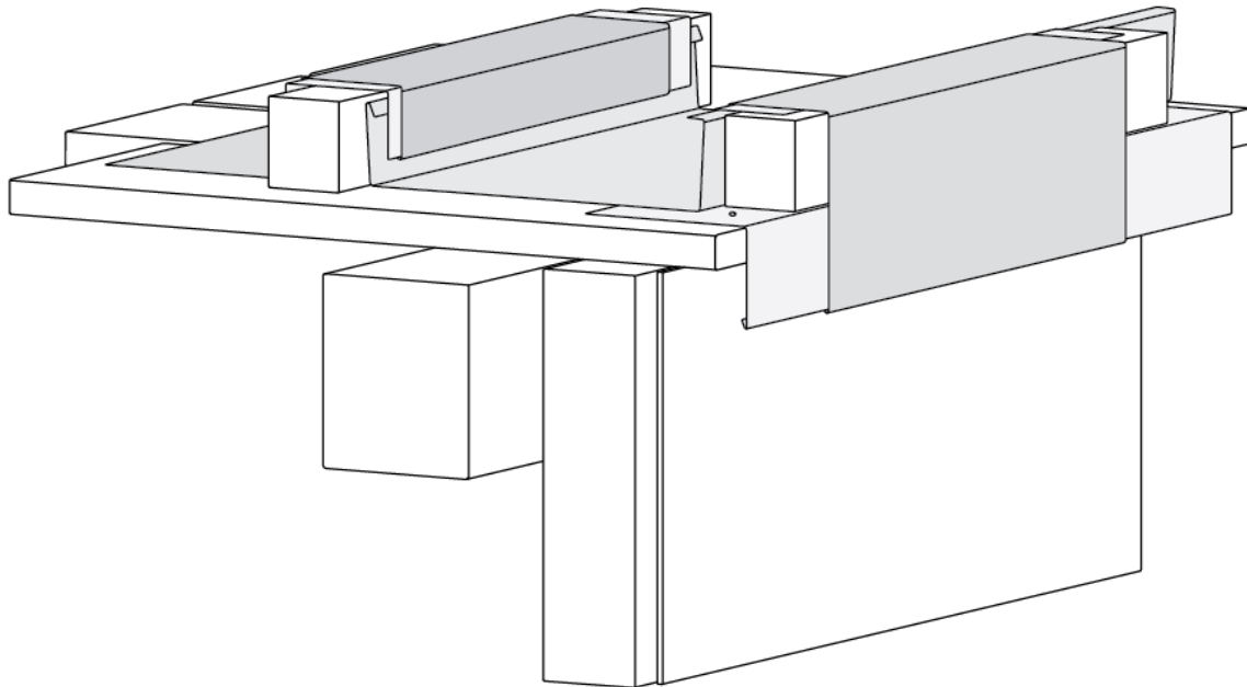
4.29 ábra A klick rendszerű lécbetétes fedés oromszegély-csatlakozása
