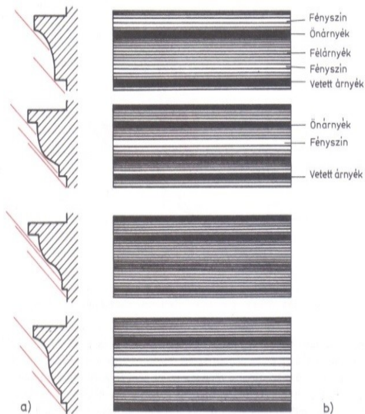
15 ábra: árnyékképzések 22
