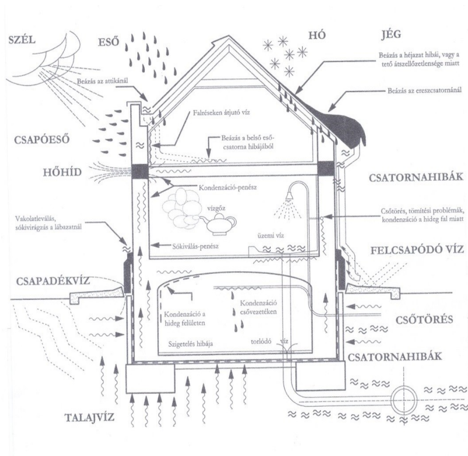
3. ábra: Szerkezetek vízterhelése 17
