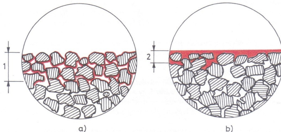
7. ábra: Impregnálószer helyes a), és helytelen b) felhordása 18
