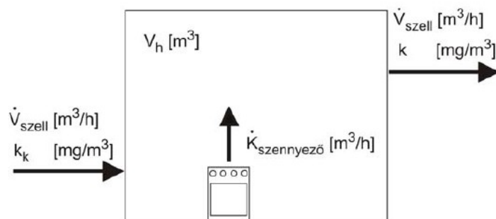
8. ábra: a számítás modellezése
