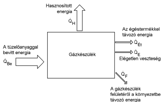
5. ábra: hagyományos gázkészülék veszteségei
