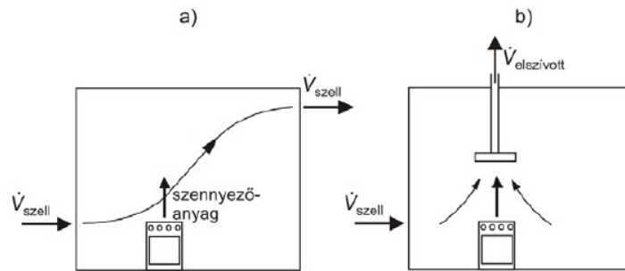
7. ábra: „A” típusú gázkészülék (a) és (b) esetben
